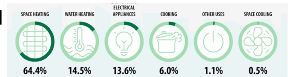
Consumo di energia nelle famiglie dell'UE. (Quota %, 2021).
